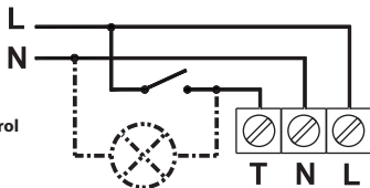
Rys.3. Higrostat (opcjonalnie), Włącznik pociągany Fig. 3. Humidistat (optional), Pull Switch Abb. 3 Hygrostat (optional), Zugschalter Рис. 3 Гигростат (опция), потолочный выключатель Obr. 3 Hygrostat (voliteľné), vupínač na šňúrku Obr. 3. Higrostat (podľa výberu), Ťahový vypínač
