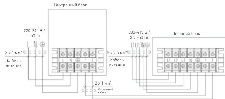
Схема электрических соединений блоков PN-36M, PN-48M, PN-60M
