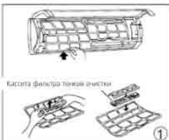
Рис. 9 Кассета фильтра тонкой очистки
