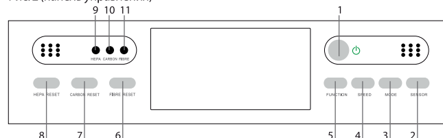
Рис. 2 (панель управления)
