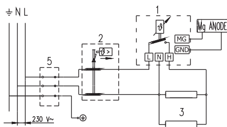
Электросхема
